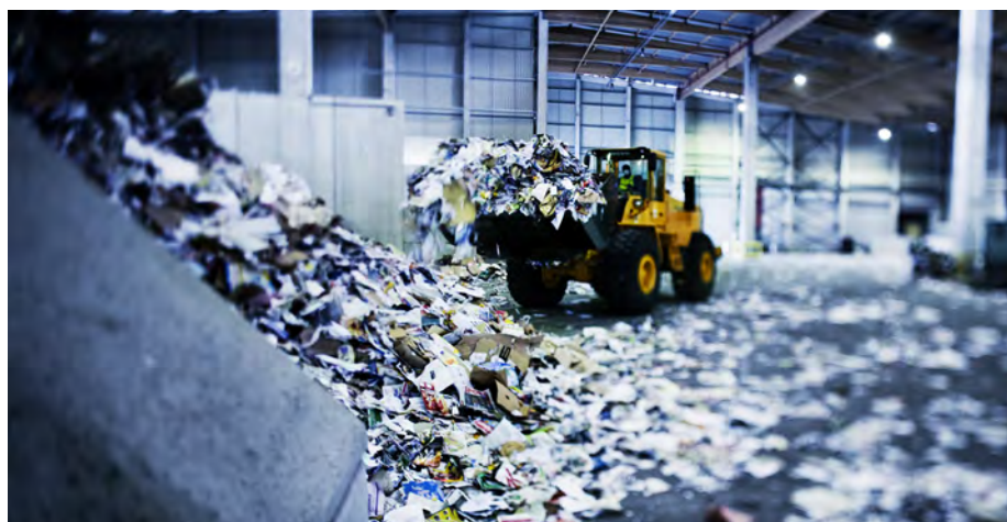
Op de sorteerlijn wordt oudpapier automatisch gesorteerd in een fractie papier en een fractie karton
